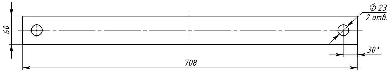
Поз.4 (Полухомут) развертка
