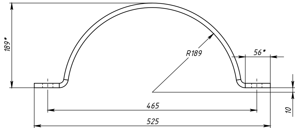
Поз.4 (Полухомут) развертка
